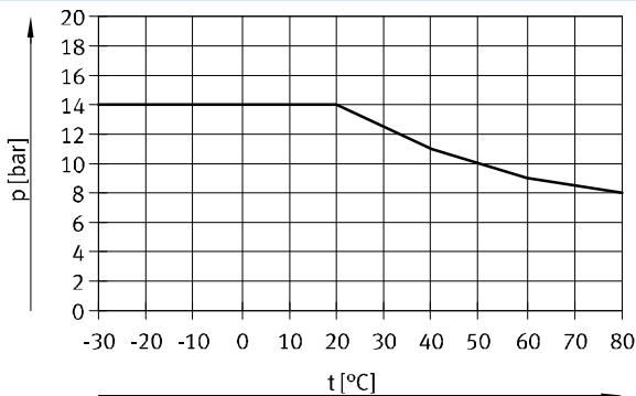
Betriebsdruck p in Abhängigkeit von der Temperatur t
