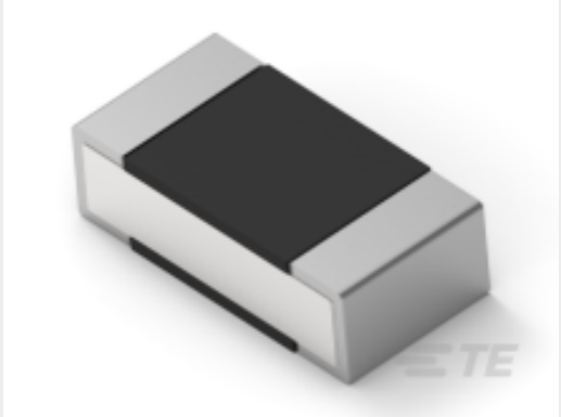
TE Part #1-2176313-5 RP 1E 0.1W 187K 0.1% 25PPM 1K RL
