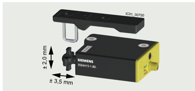
Fig. 1: Actuator tolerance
