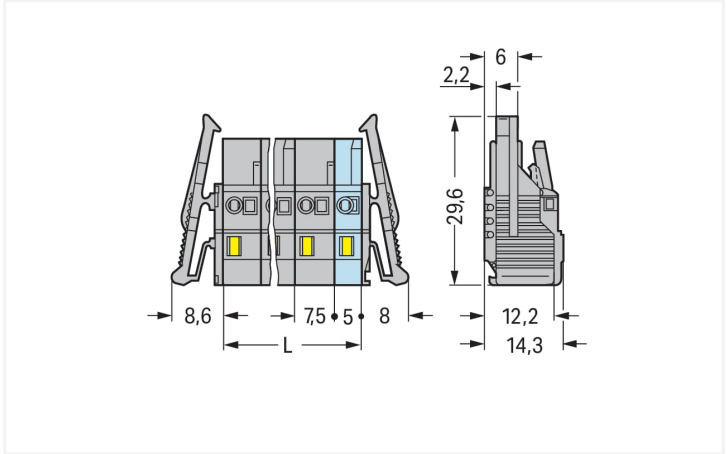
Dimensions en mm L = (Nombre de pôles – 1) x pas + 5 mm Connecteurs femelles de 2 à 3 pôles – seulement 1 crochet d'arrêt
