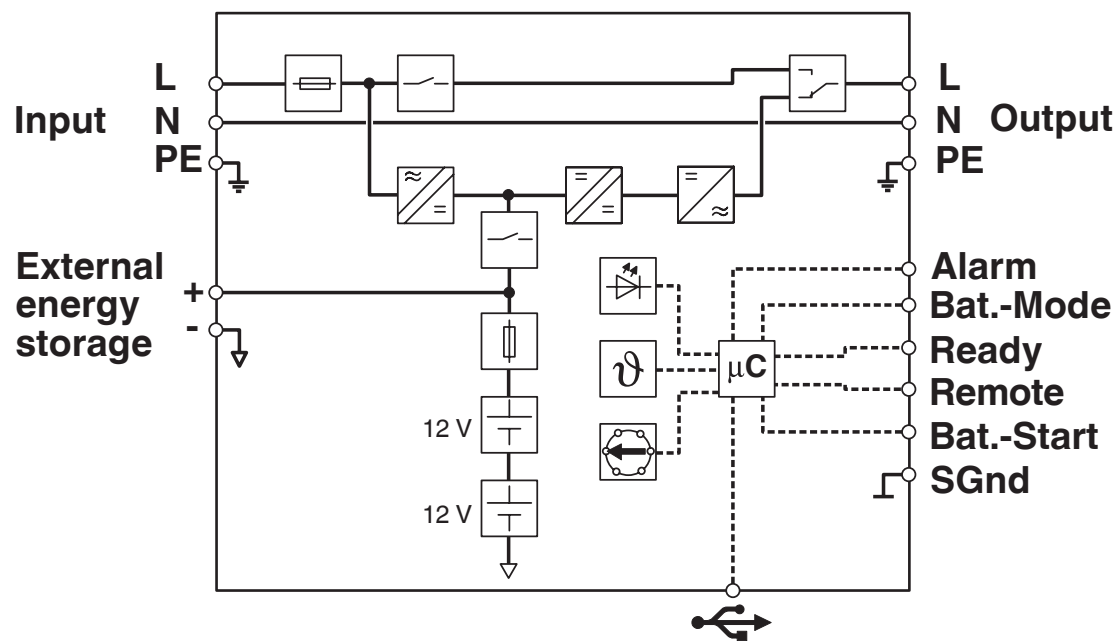
Blockschaltbild
