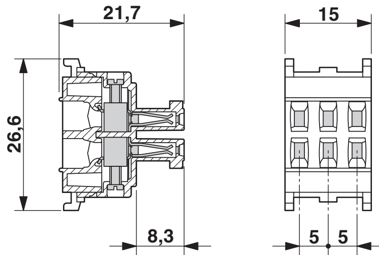
尺寸图
