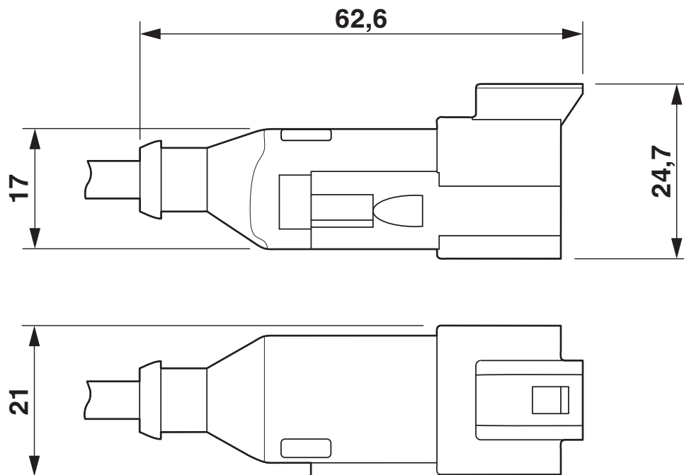
DEUTSCH DT04-3P, Drauf- und Seitenansicht
