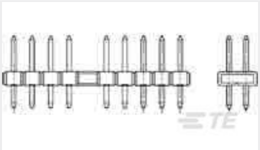
TE Part #4-5176264-8 50 AMPMODU 2MM DR VERT MNT LF
