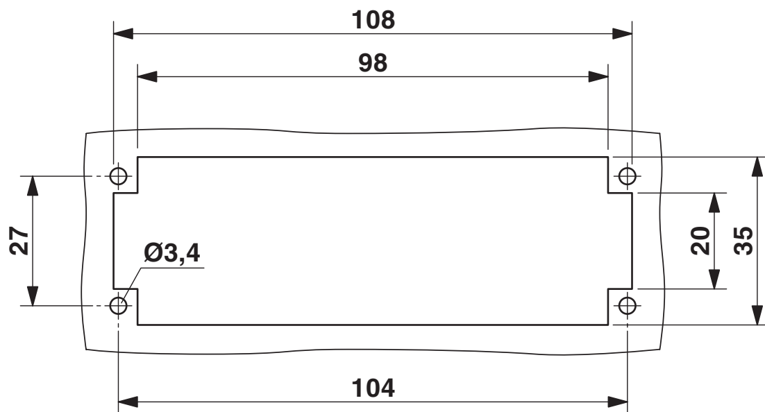
尺寸图
