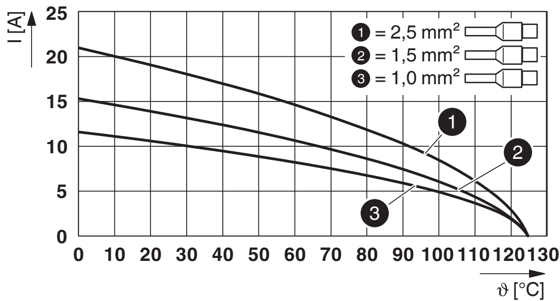
带套管柔性导线衰减曲线
