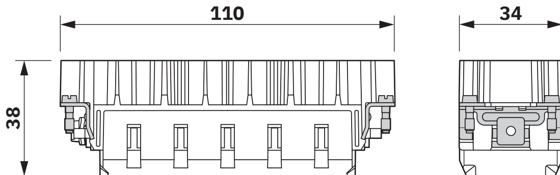
尺寸图
