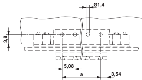
穴あけ加工図
