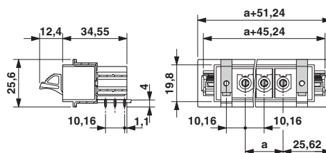
外形寸法
