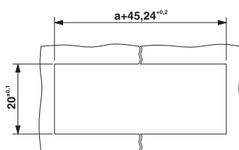
外形寸法
