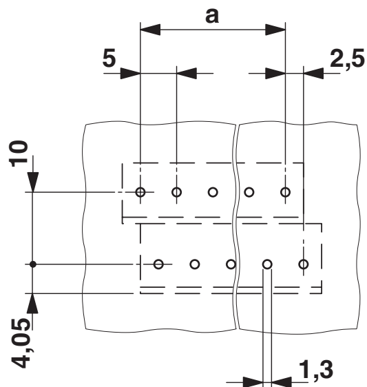
开孔图/焊盘环宽
