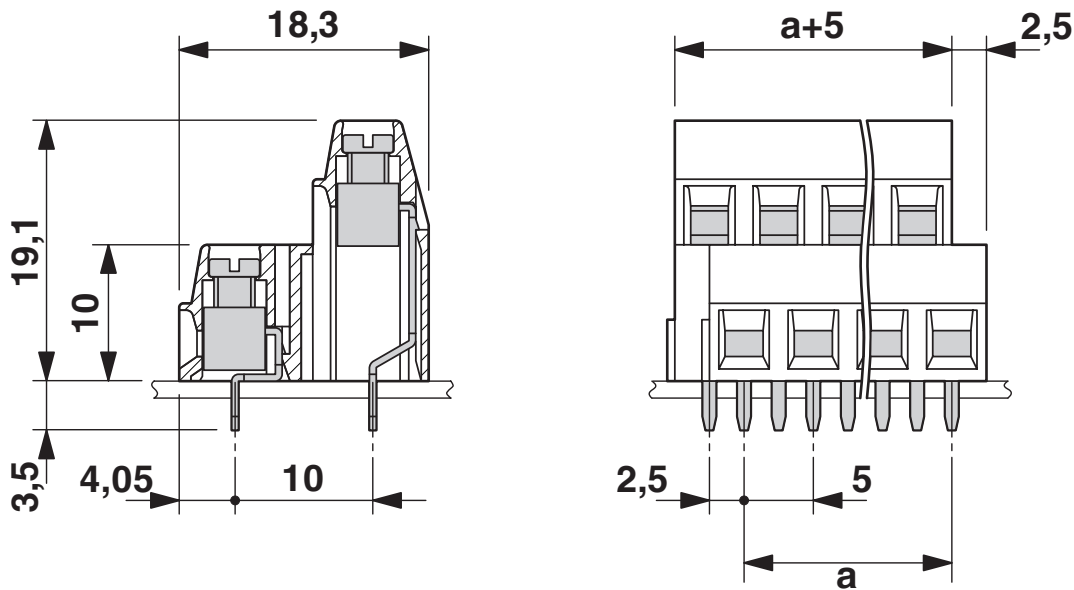
尺寸图
