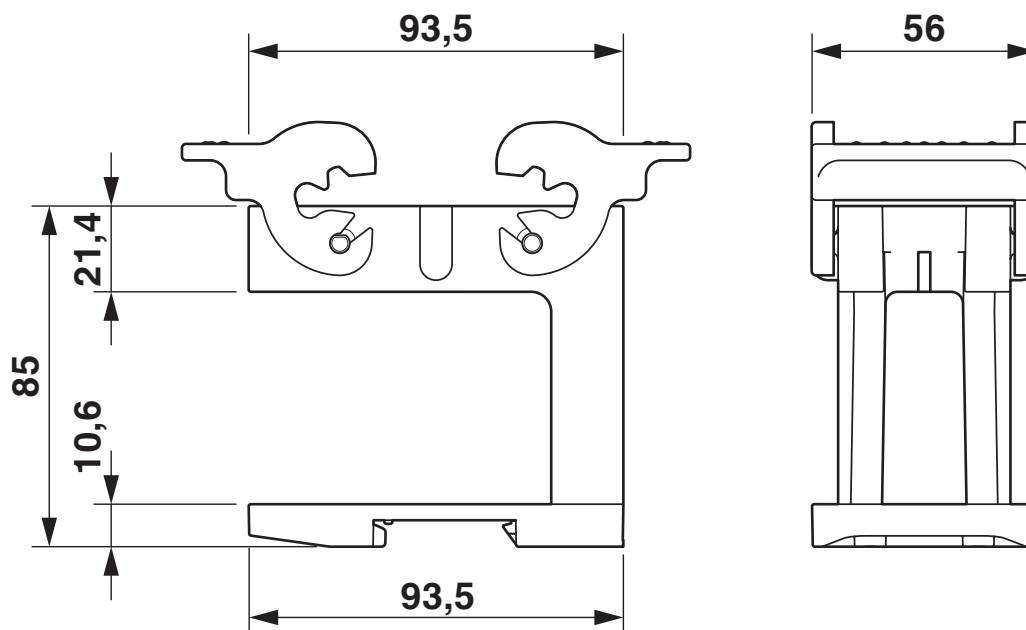
Maßzeichnung
