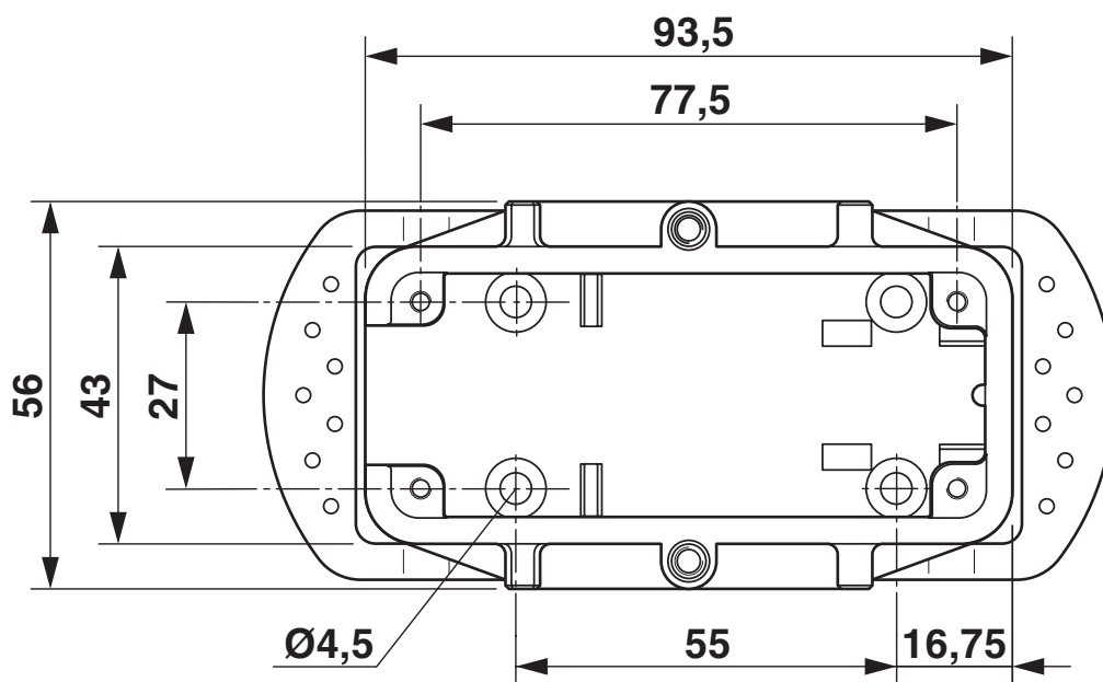
Maßzeichnung
