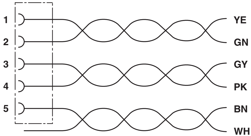
电路图
