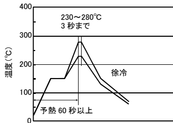
【共晶はんだ付け推奨条件】
