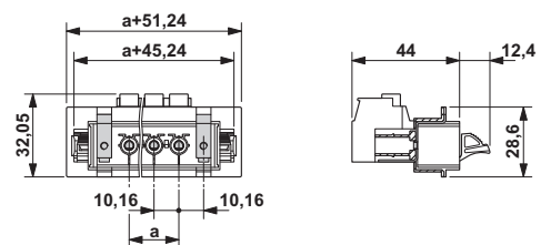
外形寸法
