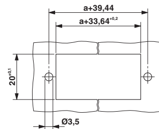
外形寸法
