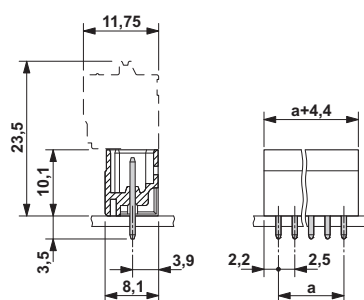
外形寸法
