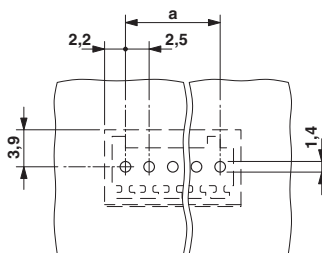
外形寸法
