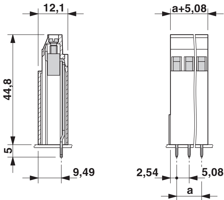
Maßzeichnung
