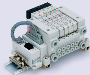
VQ1000/2000
