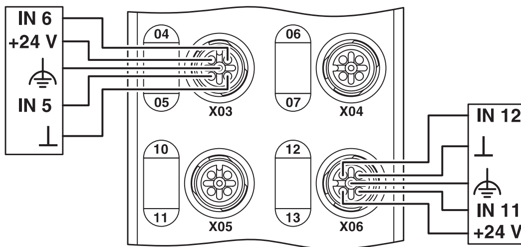
接线图
