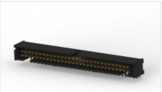
TE Part # 1-103311-2 060 LOPRO HDR RA 30DP
