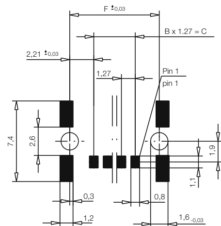
Leiterplatten-Layout Vorschlag PCB-Layout Proposal
