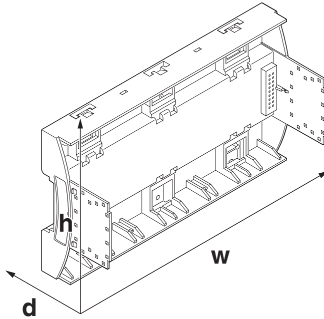
尺寸图
