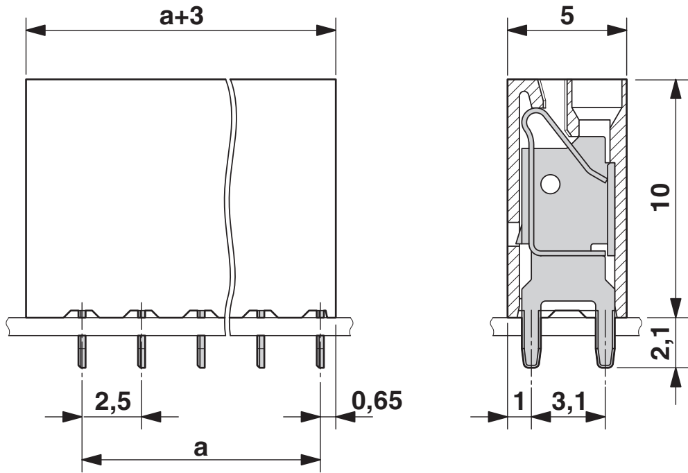
尺寸图
