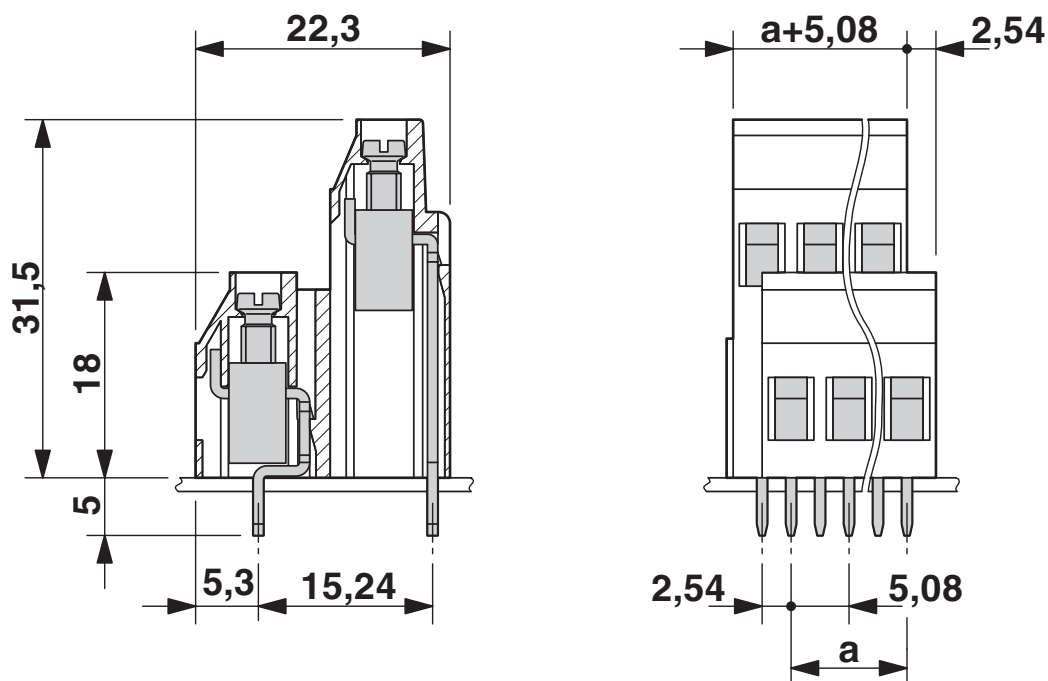
尺寸图
