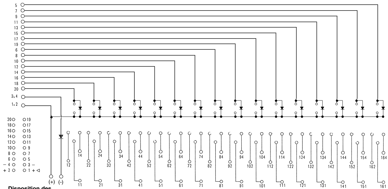
Disposition des bornes du connecteur (Vue de dessus)
