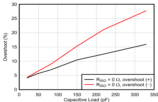
图 5-21. 小信号过冲与容性负载间的关系
