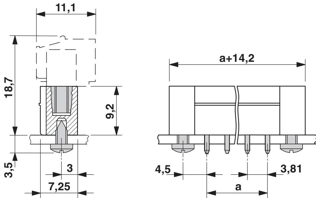
尺寸图
