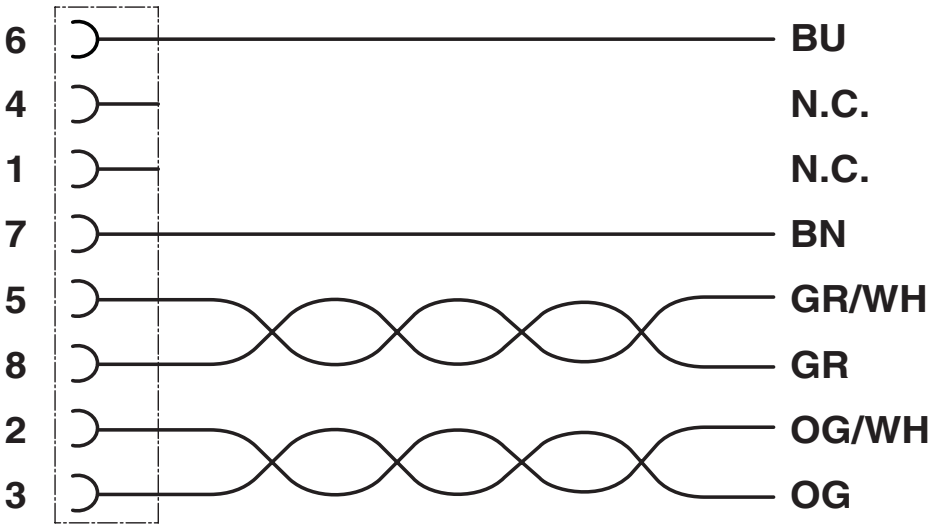
电路图
