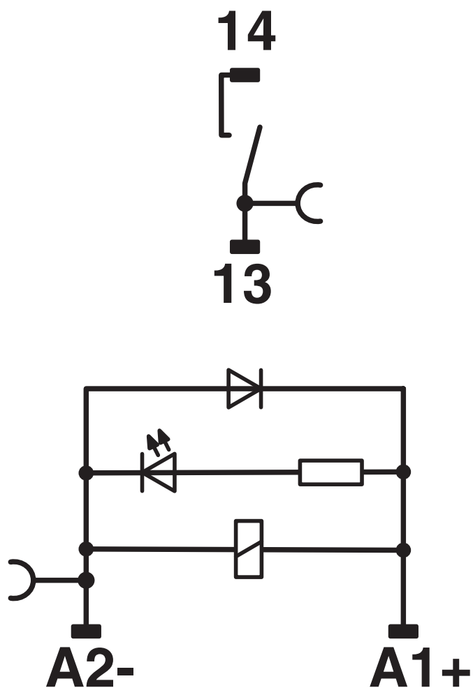
电路图
