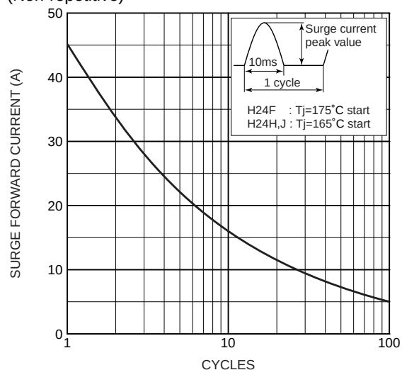
サージ順電流特性（非繰り返し） Surge forward current characteristics (Non-repetitive)
