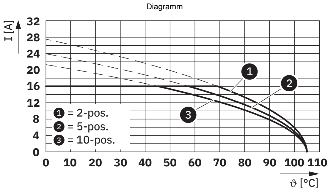
Typ: TFKC 2,5 HC/...-STF-5,08 mit CC 2,5/...-GF-5,08 P...THR
