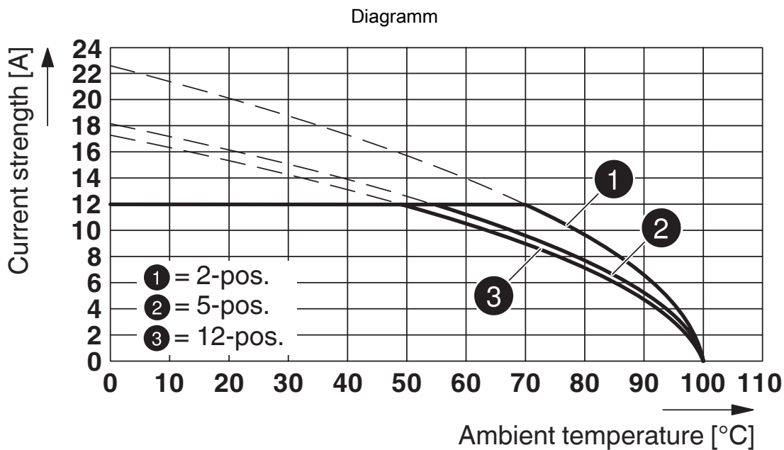
Typ: MVSTB(R/W) 2,5/...-STF-5,08 mit CC 2,5/...-GF-5,08 P26THR
