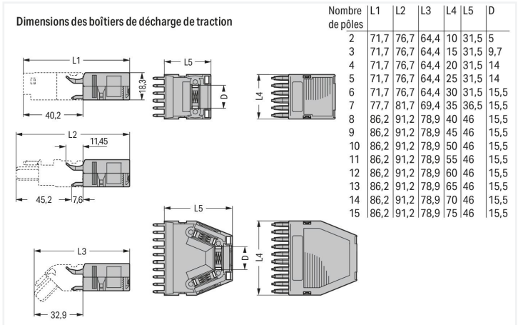
Dimensions en mm Dimensions en mm
