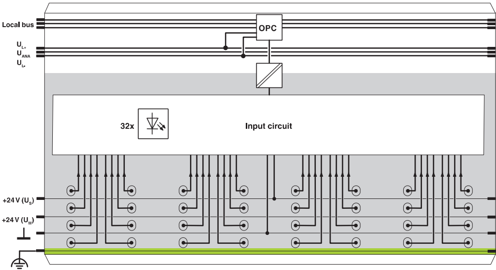
结构框图
