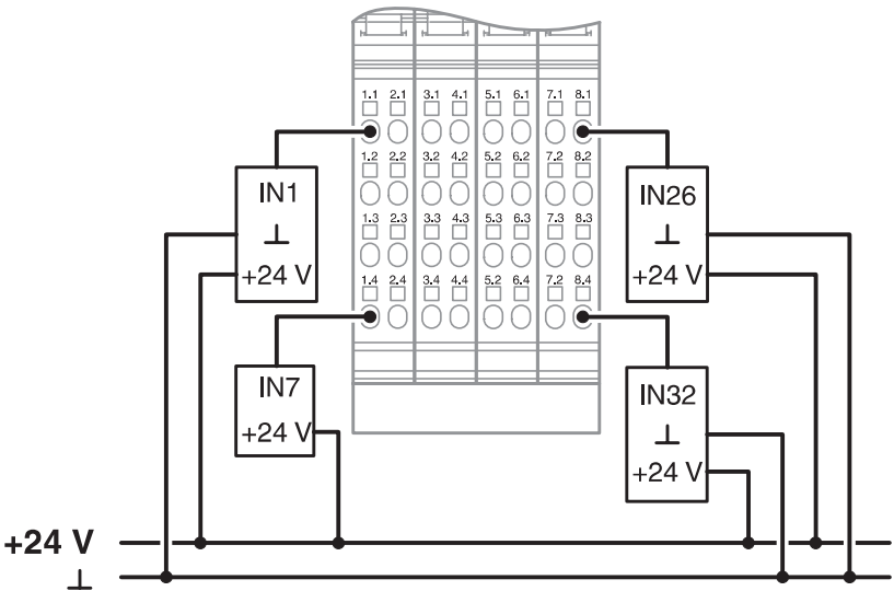
接线图
