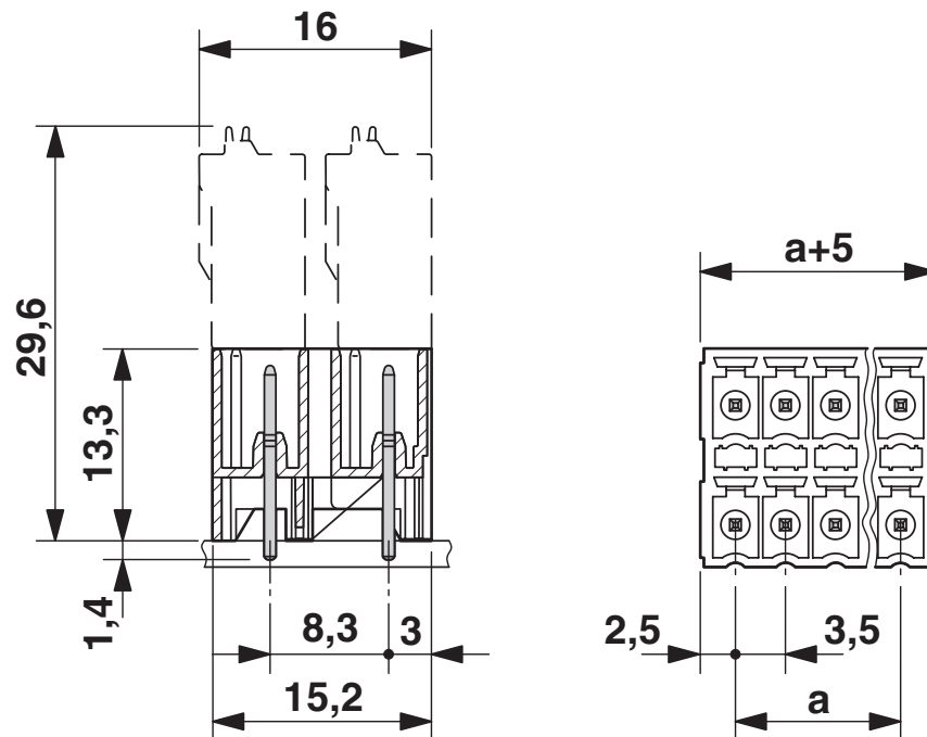
尺寸图
