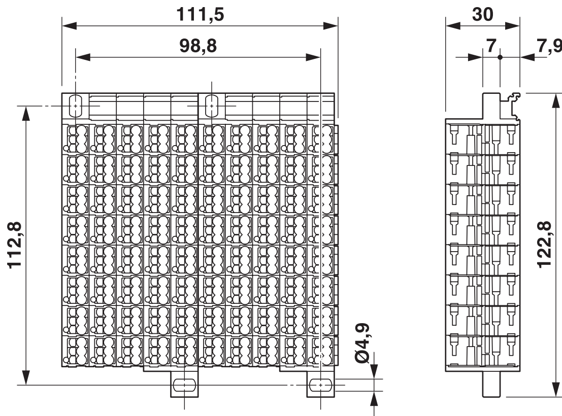
尺寸图
