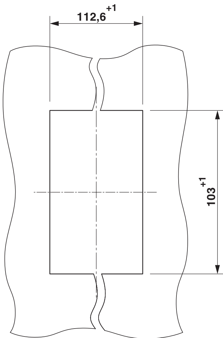
尺寸图
