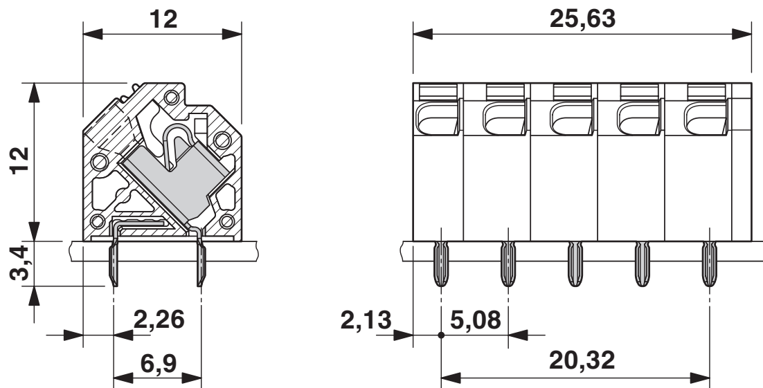
尺寸图
