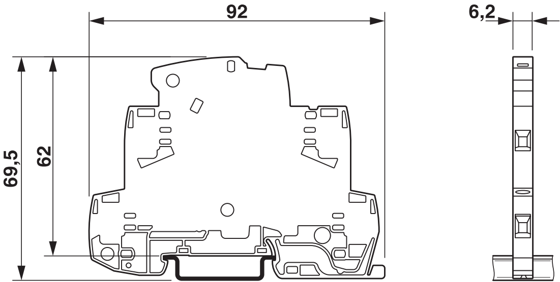
尺寸图
