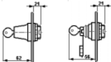
Tête de commutateur- / Tête de bouton-poussoir à clé *
