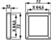
Tête d'instrument de mesure AM 72
