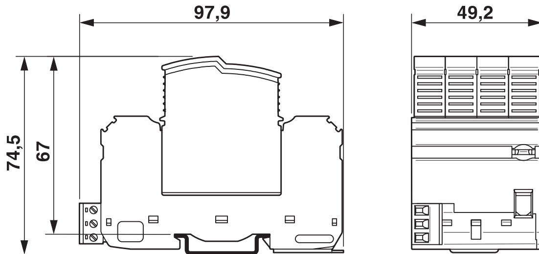
尺寸图
