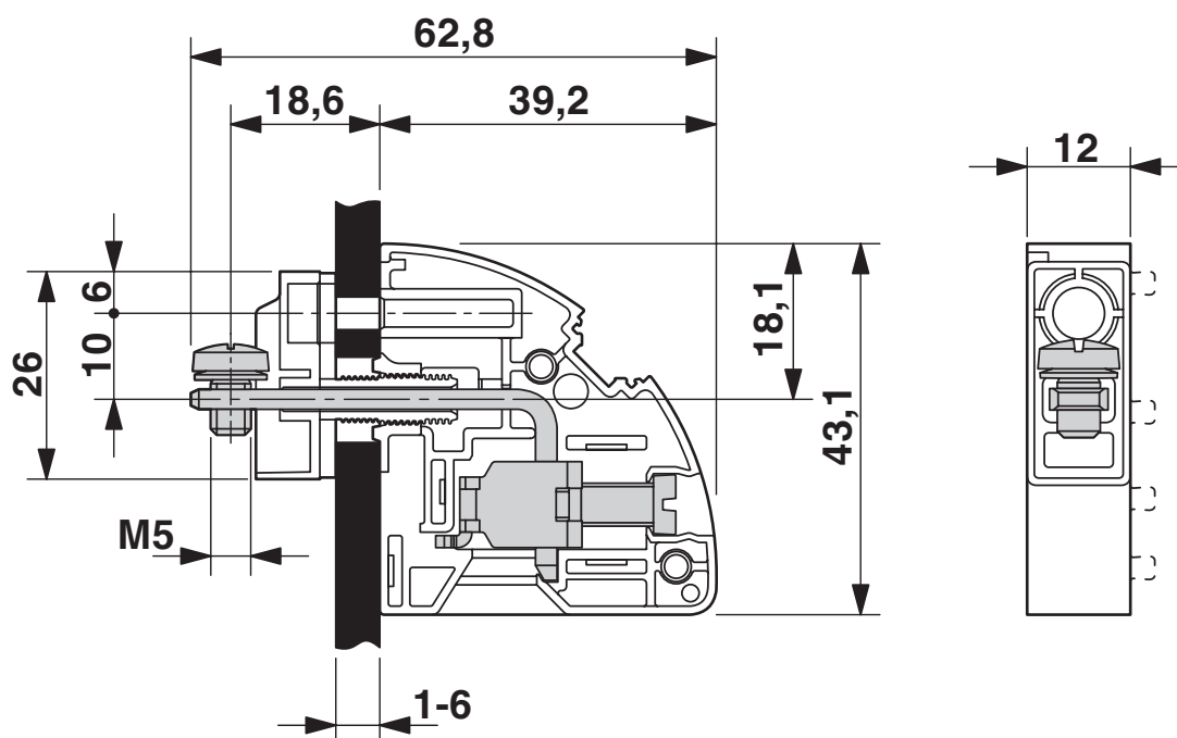
尺寸图
