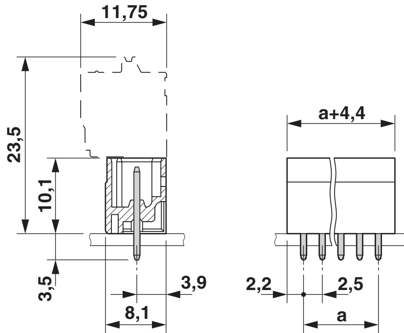
尺寸图
