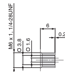
Dettagli della filettatura
