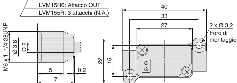
Dettagli della filettatura
