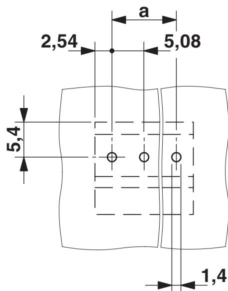
开孔图/焊盘环宽
