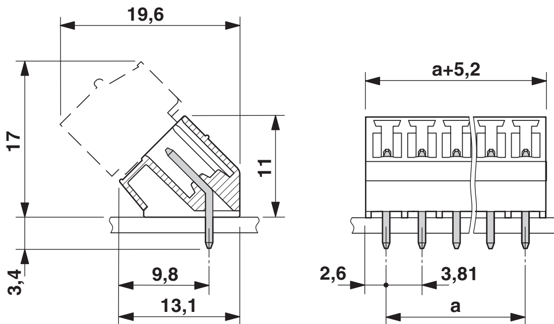
尺寸图
