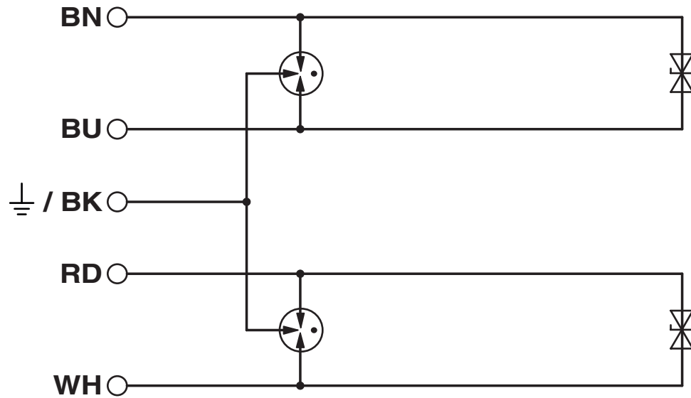
电路图
