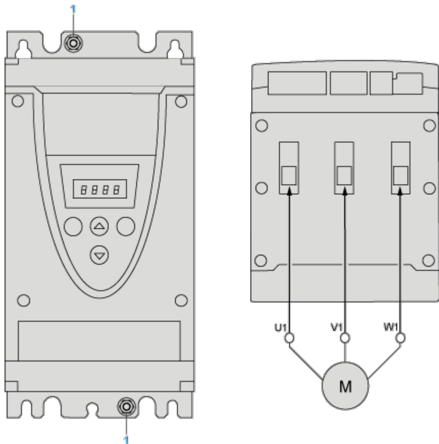
1 接地连接
