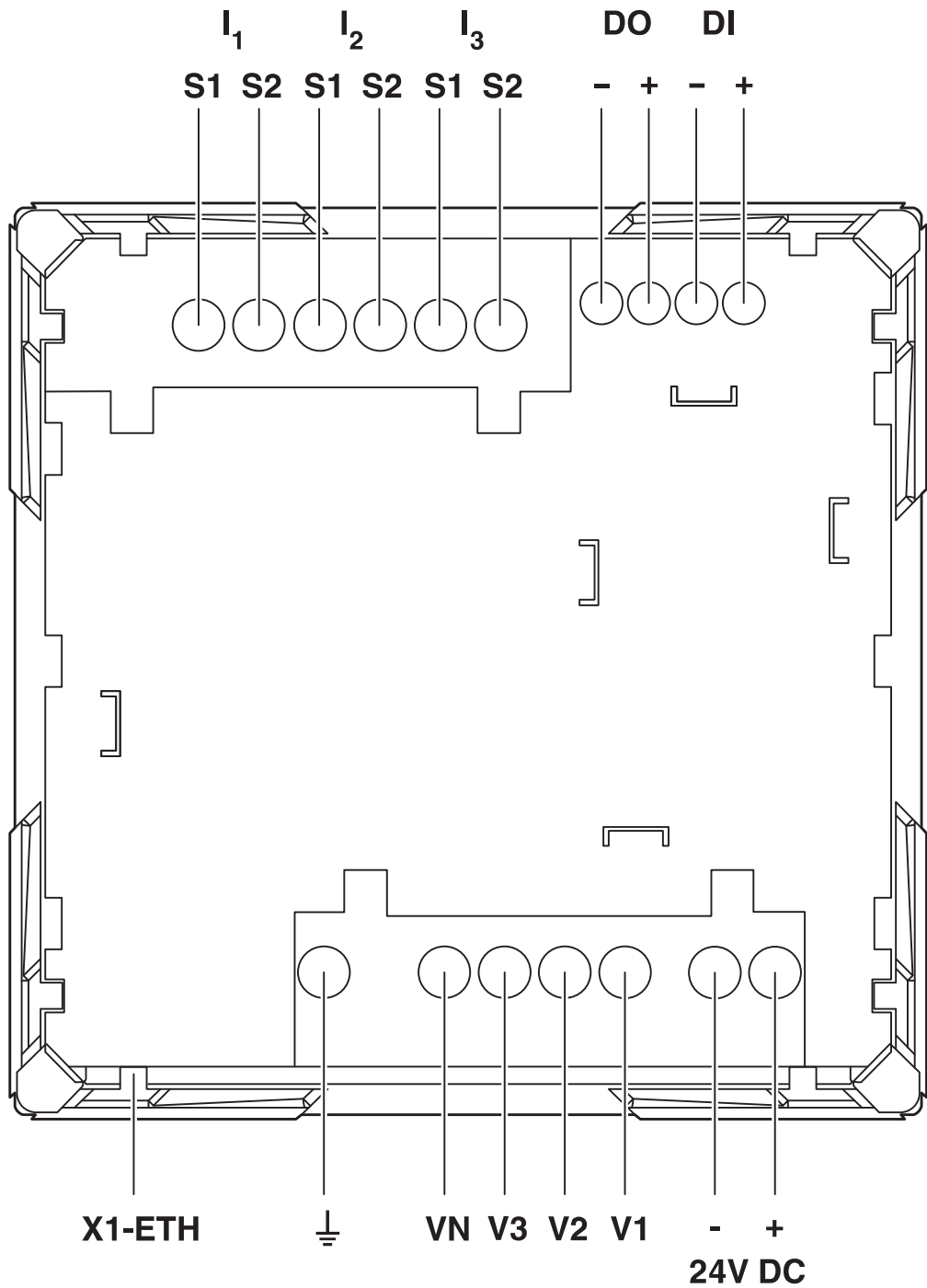
接线图
