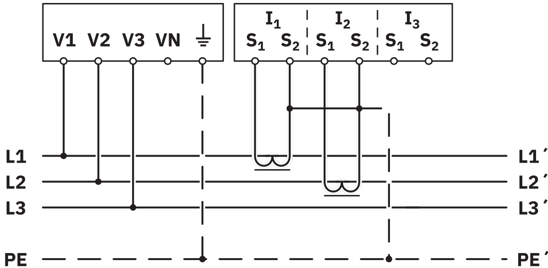
接线图
