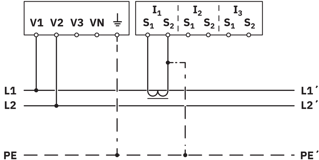
接线图
