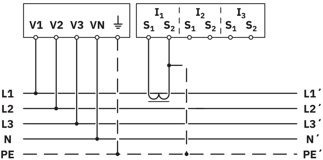
接线图
