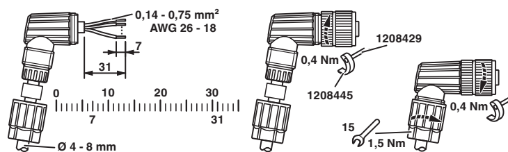
功能图
