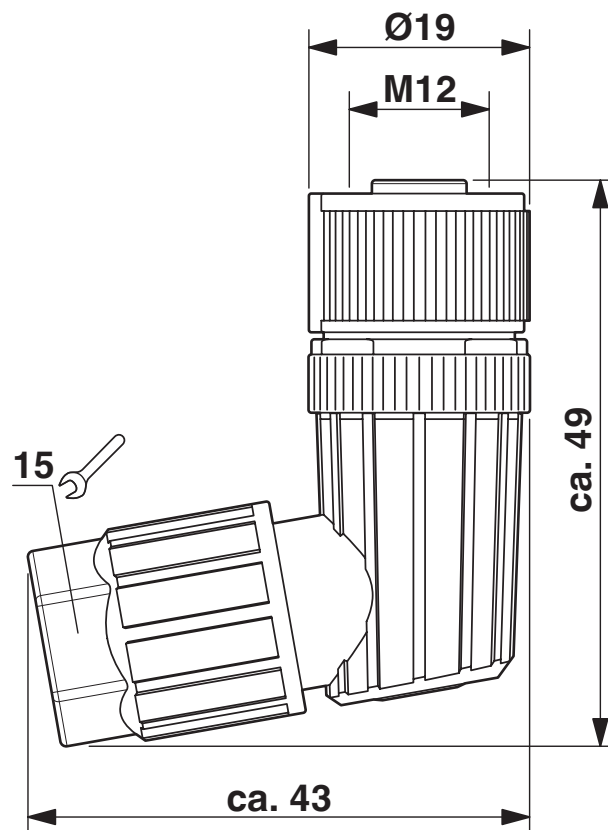
尺寸图
