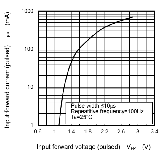
I_{FP} - V_{FP}
